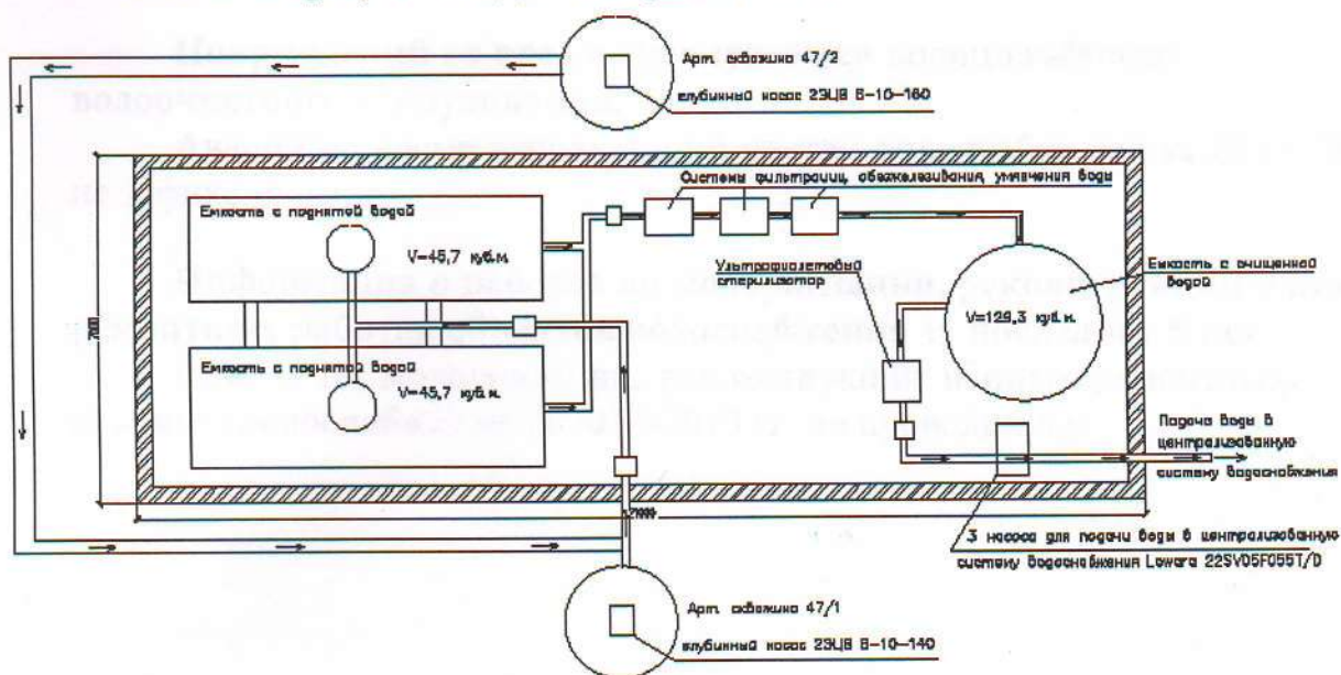
Схема технологического процесса системы водоснабжения в помещении насосной станции по адресу г. Пенза, ул. Зеленодольская, 53,63
